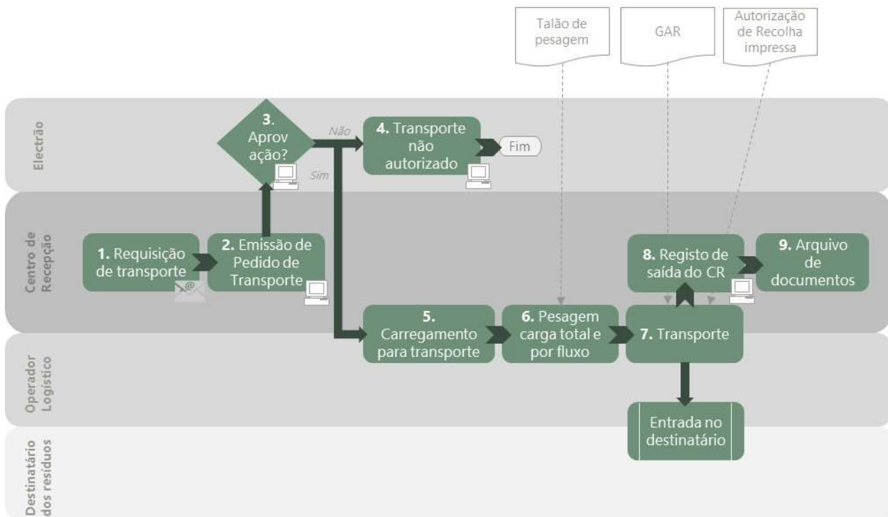
Figura 3 - Processo de expedição de REEE/RPA.
